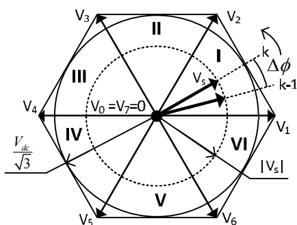
Hình 7. Phân chia đường tròn điều chế và lượng tử hóa thành phần góc quay phi
