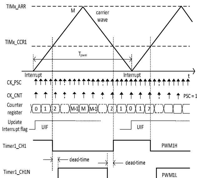
Hình 6. Giải đồ sóng của Timer1 trong chế độ PWM với sóng mang dạng tam giác cân [5]
