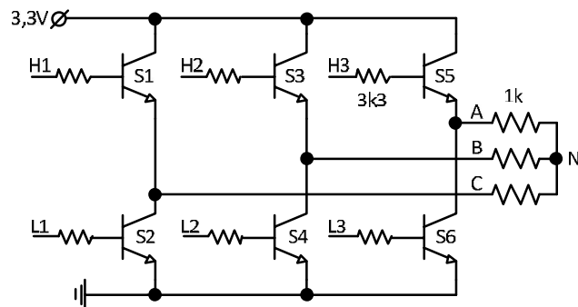
Hình 1. Mô hình thử nghiệm giải thuật điều chế biến tần ba pha hai mức SVPWM
