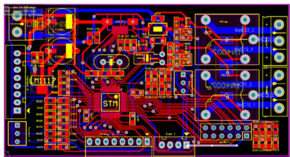
Hình 3. Bo mạch bộ điều khiển trung tâm
