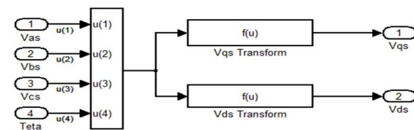
Hình 6. Khối biến đổi $V_{abc}$ sang $V_{dq}$
